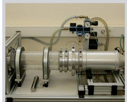
Filterprüfstand
